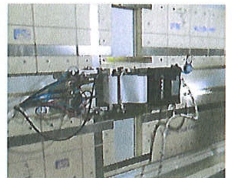
2차방벽 자동화본딩
